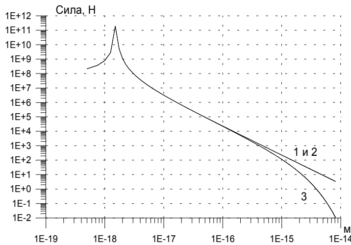
Рис.1. 1 и 2 - кулоновские и ньютоновские силы, 3 - учет потенциала Юкавы.
